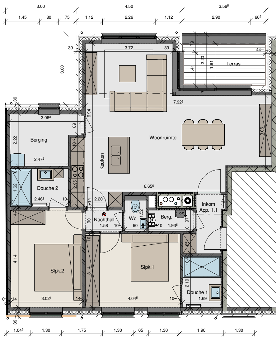
Grondplan
