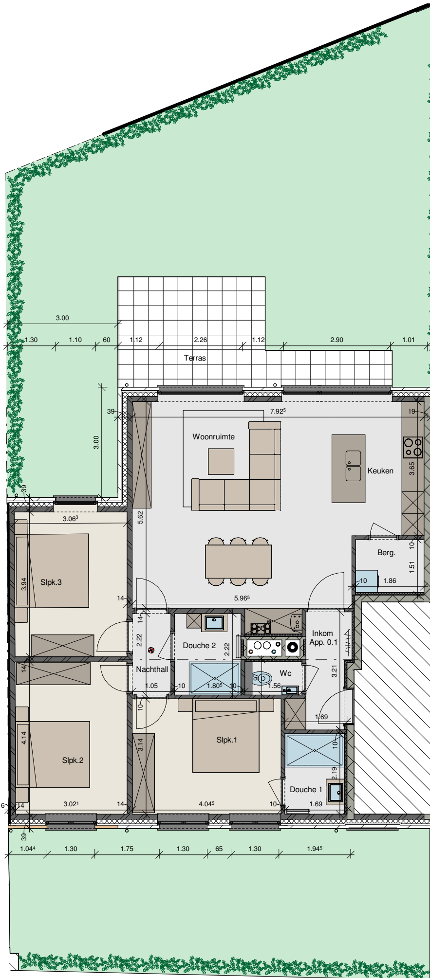
Grondplan
